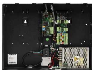
M50 kontrollerr
