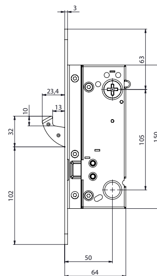
Måttitning, Connect 411-50
