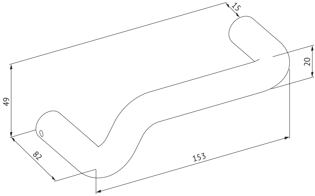
Scandinavian / DIN LH002
